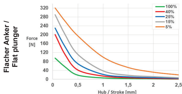
Kraft / Weg-Kennlinie Luftkühlung
